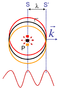
Propagation d'une onde plane
