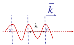
onde plane
