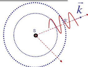
onde sphérique
