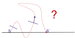
onde plane
