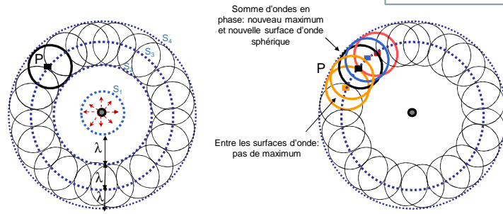
Surfaces d'ondes d'une onde sphérique
